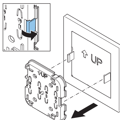
Rys. 2 - Wypnij urządzenie z zaczków płytki montażowej
