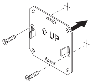
Rys. 3 - Płytkę montażową
